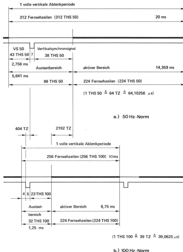
Fig. 5 Vermessung im vertikalen Ablenkbereich für beide Fernsehnormen – Définition du balayage vertical pour les deux normes de télévision
