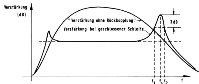
Fig. 8 Typical open- and closed-loop response Verstärkung – Gain Verstärkung ohne Rückkopplung – Gain before feedback Verstärkung bei geschlossener Schleife – Closed-loop gain
