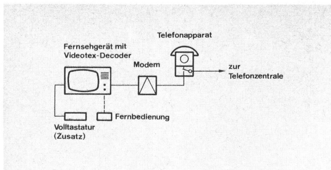
Fig. 2 Videotex-Terminal – Terminal Videotex Fernsehgerät mit Videotex-Decoder – Téléviseur avec décodeur Video- tex Telefonapparat – Appareil téléphonique Zur Telefonzentrale – Vers le central téléphonique Volltastatur (Zusatz) – Clavier complet (en supplément) Fernbedienung – Télécommande
