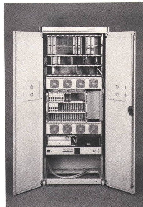
Fig. 3 EMX 1010, grosses System (Schranktüren geöffnet). Von oben nach unten Rechner- und Speichereinschübe, Leitungsanschlusseinheiten, Speisung und Floppy-disk-Laufwerk — Grand système EMX 1010 (portes ouvertes). De haut en bas le calculateur et les unités enfichables de mémorisation, les unités de connexion de ligne, l'alimentation et l'unité du disque souple
