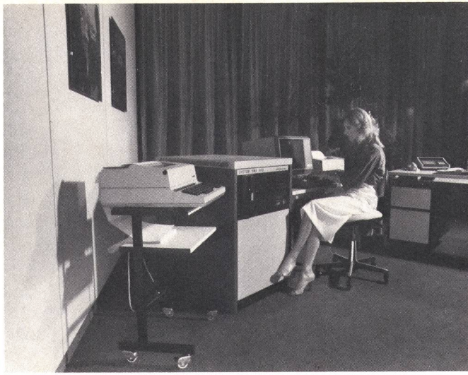
Fig. 2 EMX 1010, kleines System. Von links nach rechts Journalmaschine, Systemschrank, Vermittlerplatz — Petit système EMX 1010. De gauche à droite, l'imprimante du journal, l'armoire abritant des systèmes, la position de commutation
