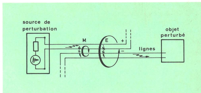
Fig. 6 Couplage par des champs rapprochés électriques et magnétiques M Champ magnétique E Champ électrique Signal perturbeur
