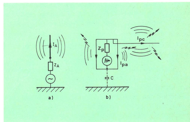
Fig. 7 Rayonnement a Antenne «réelle», le courant d'antenne ( I_A ) produit le rayonnement b Courant perturbateur circulant dans l'appareil ou dans le câble faisant office d'antenne Z_A Impédance d'antenne I_A Courant d'antenne I_{pa} Courant induit sur les parties métalliques de l'appareil I_{pc} Courant induit sur le câble raccordé Signal perturbeur
