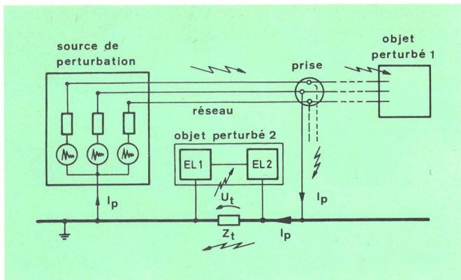
Fig. 5 Perturbations transmises par conduction Objet perturbé 1 est directement influencé par les conducteurs du réseau Objet perturbé 2 est perturbé par la chute de tension U_t dans un système de terre non idéal (impédance de terre Z_t \neq 0 ; les circuits électroniques 1 et 2 sont reliés par une ligne de transmission de signaux et sont mis à la terre en différents points) EL 1, 2 Circuit électronique I_p Courant de la source de perturbation Z_t Impédance du conducteur de terre U_t Tension perturbatrice apparaissant dans le conducteur de terre Signal perturbeur
