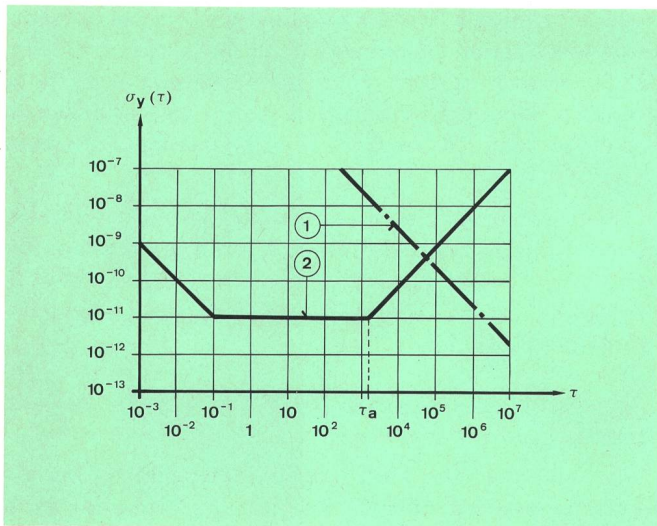
Fig. 3 Stabilitätsdiagramm \sigma_y(\tau) eines Quarzoszillators — Diagramme de stabilité \sigma_y(\tau) d'un oscillateur à quartz ① Bedingung — Condition \sigma_y(\tau=t) \cdot t = 1,9 \cdot 10^{-5} ② Quarzoszillator — Oscillateur à quartz \sigma_y(\tau) Allan-Varianz der relativen Frequenzabweichung y(t) — Variance d'Allan de la déviation relative de fréquence y(t) \tau Betrachtungsintervall — Intervalle d'observation \tau_a Grenze oberhalb welcher \sigma_y(\tau) durch Alterung bestimmt ist — Limite au-dessus de laquelle \sigma_y(\tau) est déterminée par le vieillissement
