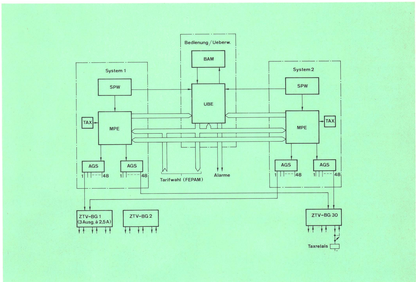
Fig. 5 Systemkonzept des nationalen Zeittaktgebers NZG 731
