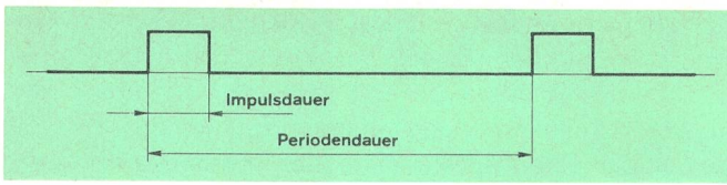
Fig. 6 Begriffe bei Impulsfolgen
