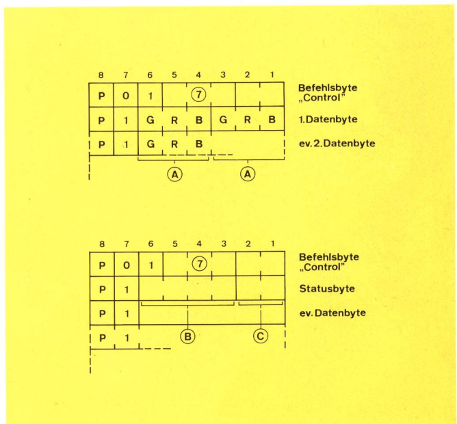
Fig. 15 Aufbau der Bildsteuerbefehle — Structure des instructions de commande d'image (A) Farb- und Helligkeitswerte mit abnehmender Intensität — Valeurs de chrominance et de luminosité par intensité décroissante (B) Spezifikationsfeld — Secteur de spécification (C) Ergänzungsfeld — Secteur de complément Befehlsbyte «Control» — Byte d'instruction «Control» Datenbyte — Byte de données Statusbyte — Byte d'état
