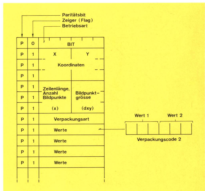
Fig. 20 Format der fotografischen Bildübertragung beim Telidon-System — Format de la transmission photographique d'images dans le système Telidon Paritätsbit — Bit de parité Zeiger (Flag) — Élément d'identification (Flag) Betriebsart — Mode d'exploitation Koordinaten — Coordonnées Zeilenlänge, Anzahl Bildpunkte — Longueur des lignes, nombre de points d'image Bildpunktgrösse — Grandeur des points d'image Verpackungsart — Mode d'assemblage Werte — Valeurs Verpackungscode — Code d'assemblage
