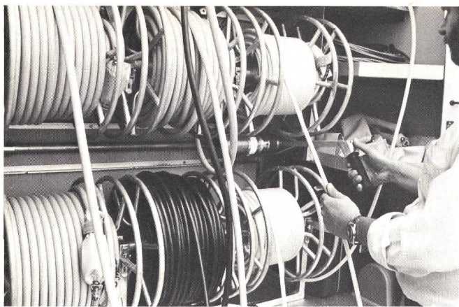
Fig. 6 Kabelrollengestell mit den sechs elektrisch angetriebenen Kabelrollen — Bâti de tambours de câbles, dont six sont actionnés par un moteur électrique
