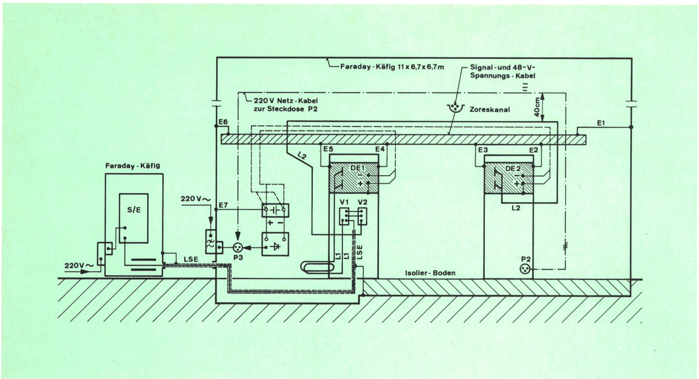
Fig. 1 Versuchsaufbau mit zwei IFS-Durchschalteeinheiten (DE1-DE2) V1-V2 Kabelverteiler L1-L2 VF-Signalkabel 2 x (16 x 4), zwischen DE1-V1 beziehungsweise DE2-V2
