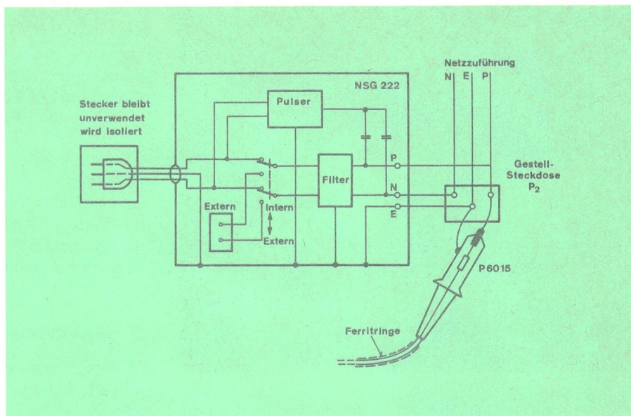
Fig. 11 Störgenerator NSG 222 als störender Verbraucher betrieben (Störspannung asymmetrisch) Die Sonde P6015 blieb für alle Messungen stets an den Ausgangsbuchsen angeschlossen, auch wenn das Kathodenstrahloszilloskop nicht angeschlossen war
