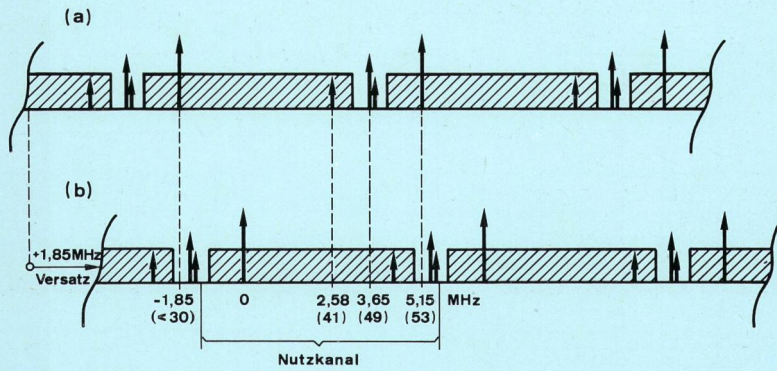
Fig. 2 Kanalraster a) CCIR-Standardraster für den Bereich III, Norm B
