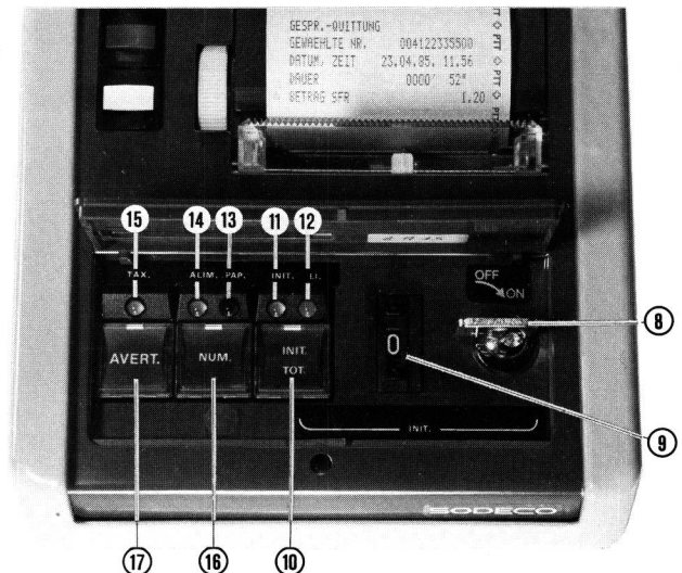
Fig. 4 Steuer- und Kontrollelemente – Organes de commande et de contrôle
