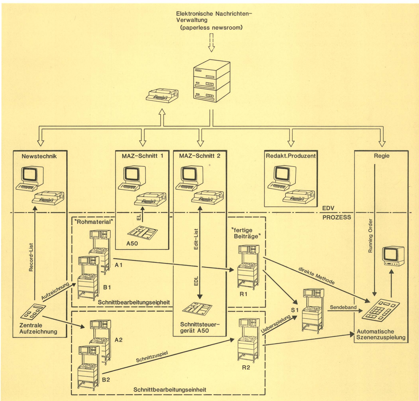
Fig. 7 Betriebskonzept MAZ-System
