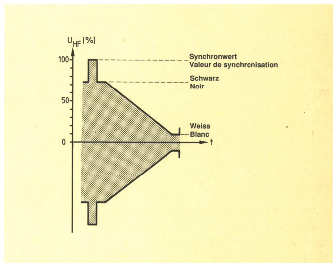
Fig. 4 TV-Signal-Hüllkurve – Enveloppe du signal TV
