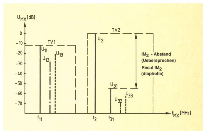
Fig. 3 Übersprechen TV1 nach TV2: Vereinfachtes Modell der Intermodulation 2. Ordnung – Diaphotie TV1/TV2: modèle simplifié d'une intermodulation du 2 e ordre Erläuterungen im Text – Explications dans le texte
