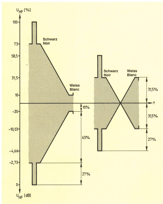
Fig. 6 Hüllkurven-Darstellung des normgerecht modulierten TV-Signals (links) und des trägerreduzierten TV-Signals im endgültigen Arbeitspunkt (rechts) – Représentation de l'enveloppe du signal TV modulée selon la norme (à gauche) et du signal TV à porteuse réduite au point de fonctionnement définitif (à droite)
