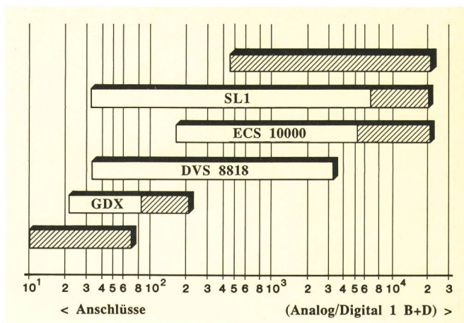
Fig. 32 PTT-Angebot digitale TVA – Offres des PTT en ECA numériques Anschlüsse – Raccordements (analog/digital 1B + D) – (analogique/numérique 1B + D) In Vorbereitung – En préparation
