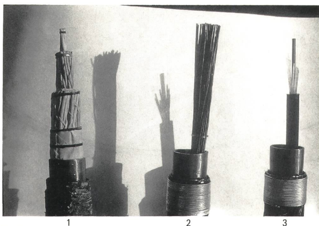
Fig. 1 Darstellung der Auswirkung des Ausbrennvorganges 1 DM-Papierlufttraumkabel 3 Eingezogenes Glasfaserkabel 2 Ausgebranntes Kupferbündel
