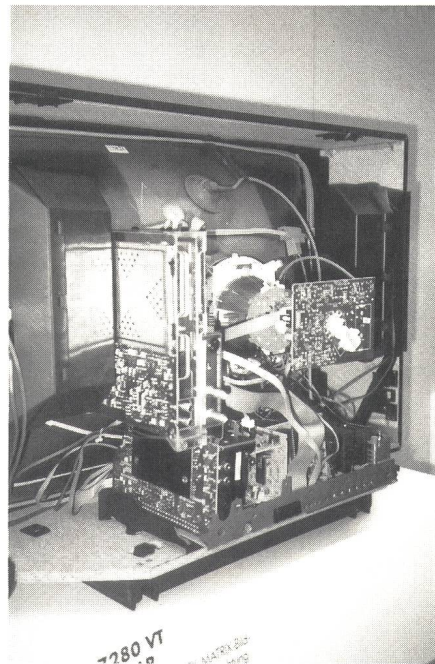
Fig. 10 TV-Empfänger von Saba mit eingebauten Decodern für den Empfang von TV-Signalen des ECS-Satelliten und für D2-MAC des TV-Sat 1 (Foto Autor)
