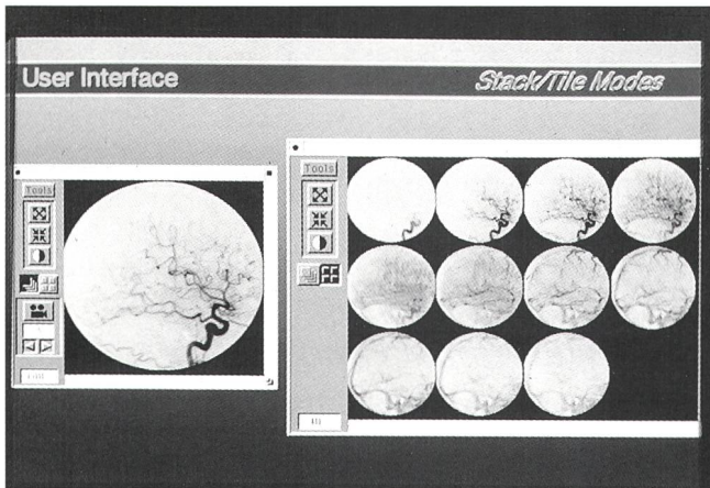
Fig. 6 Beispiel einer dynamischen Untersuchung an Blutgefäßen des Gehirns (zeitliche Abfolge angiographischer Aufnahmen nach Injektion von Kontrastmittel)
