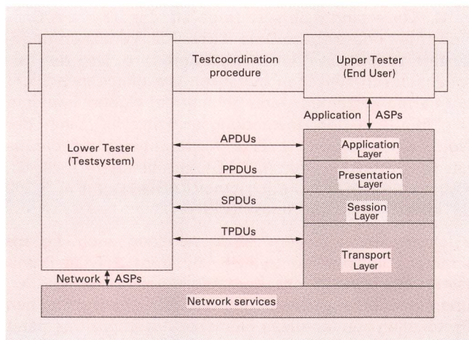
Fig. 6 Entferntes Einschichten-Testen
