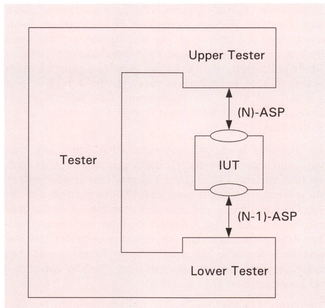
Fig. 5 Testkonzept
