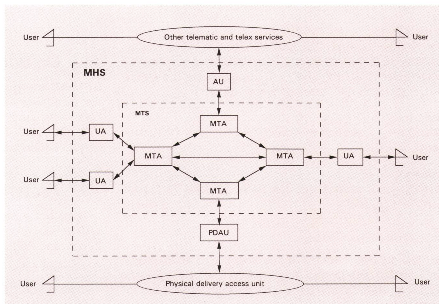
Fig. 2 Funktionales Modell MHS
