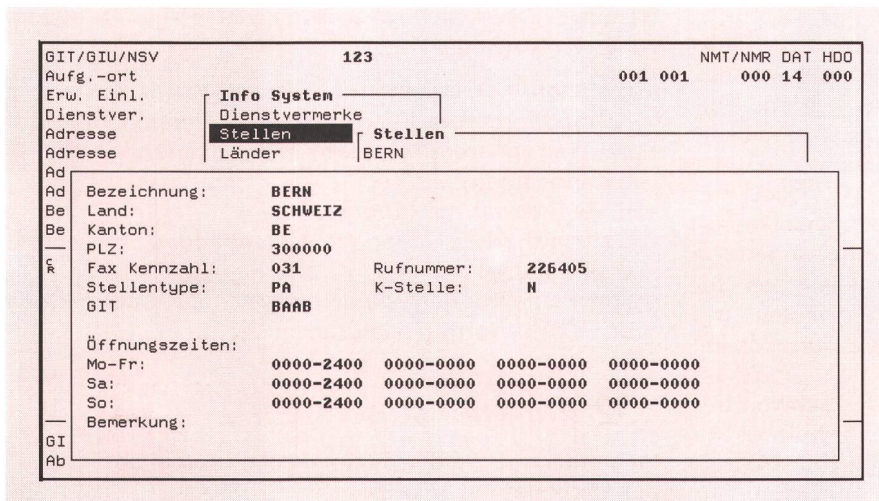
Fig. 5 Bildschirmmaske
