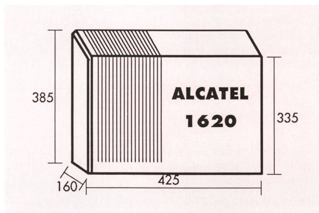
Fig. 3 Gehäuseabmessungen
