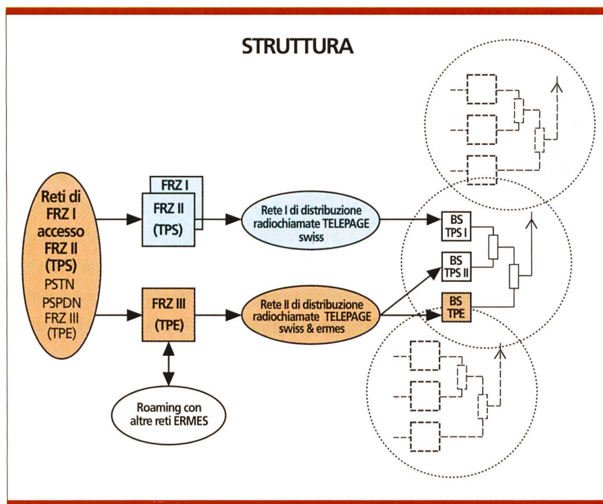
Fig. 3. Struttura del sistema TELEPAGE ERMES.
