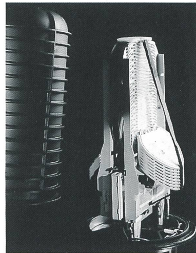
Kompakte Muffenausführung
