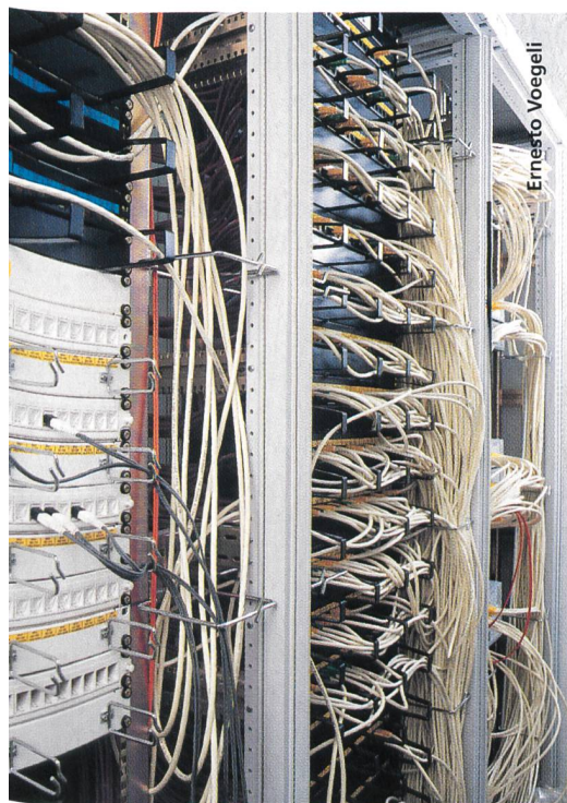
Bild 3. Verkabelung.
