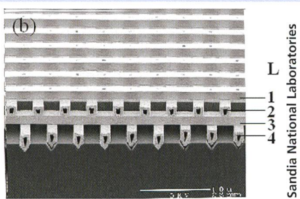
Dreidimensionales Wolframkristall.
