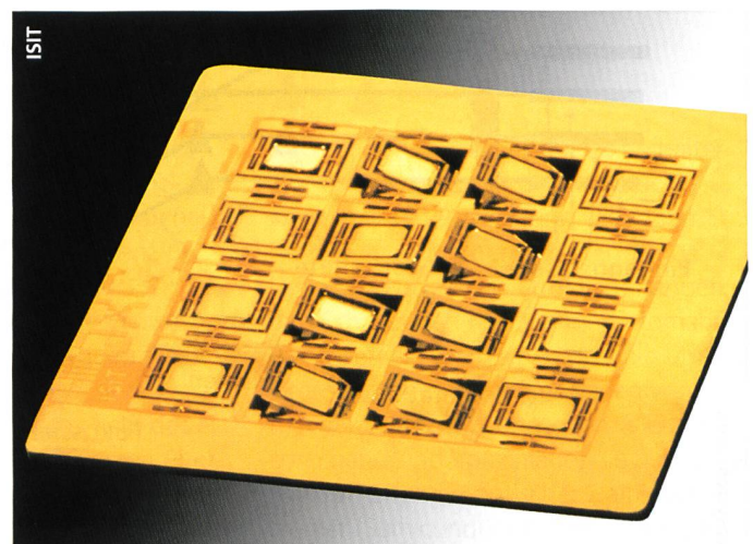
Bild 4. Zweiachsen-Kippspiegel-Matrix.
