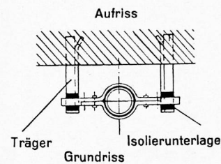
Abbildung 3 Beispiele für Isolierte Rohr- befestigungen a. d. Gebäudekonstruktion
