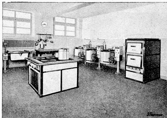
THERMA-Grossküche in der Anstalt Viktoria, Wabern
