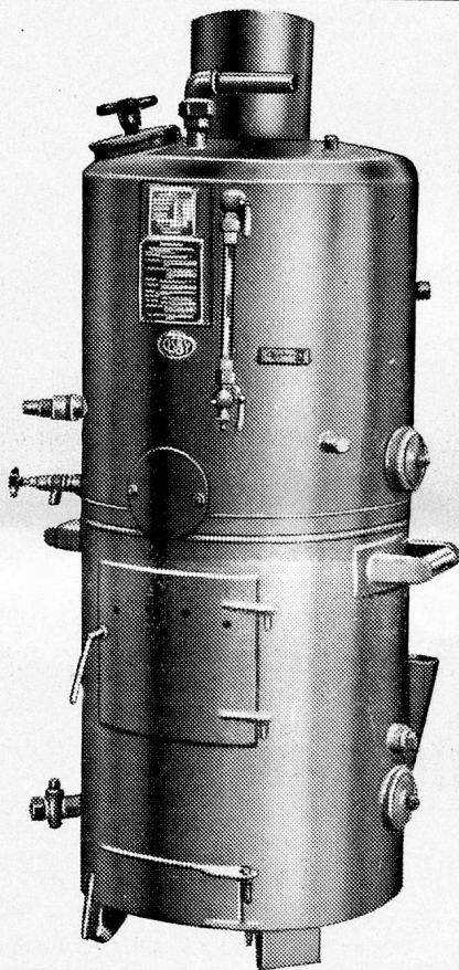
Der Osby-Kessel wird in 14 verschied. Grössen gebaut. (Das Bild zeigt Type 2.)
