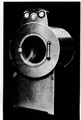
Wäsche-Tumbler (Wäschetrockner) 45 kg Trockenwäsche pro Stunde
