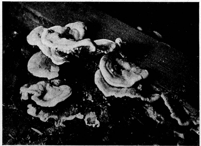
Zerstörung eines Bodenbalkens durch den echten Hausschwamm
