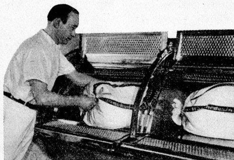
Die verschlossenen Säcke werden in die Maschine geladen
