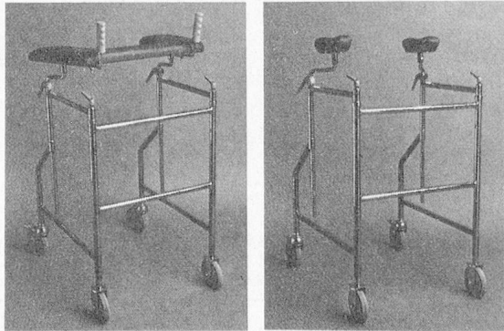
Gehwagen mit Armauflage (Abb. links) und Achselstützen (Abb. rechts) Lenkrollen mit Doppelstopp, höhenverstellbar, gepolstert mit Kunstlederbezug, zusammenlegbar mit wenigen Handgriffen, lässt sich bequem in jedem Kofferraum mitführen.
