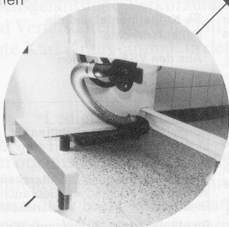
Dank elektro-Linearantrieb günstige Masse. Totale Länge ab Wand = 200 cm kurze Füße für optimale Bodenfreiheit
