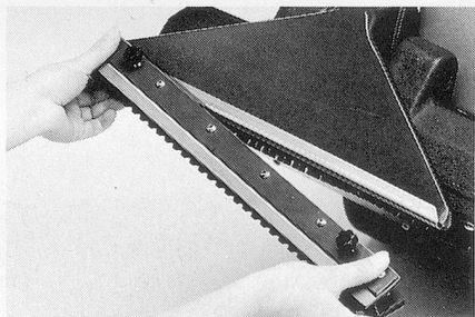
Spezielle Hartbelagsdüse.
