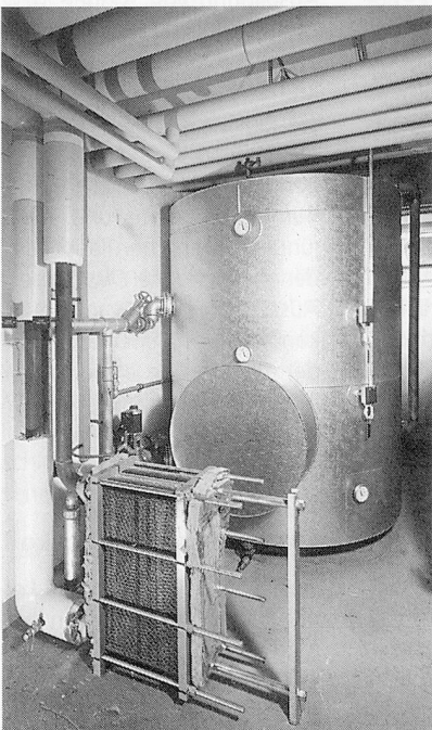
Der bestehende Boiler wurde neu isoliert; er wird nun über einen Plattenwärmetauscher (vorne, offen) vom Kessel mit Wärme versorgt.
