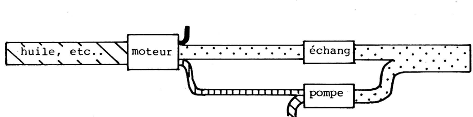
POMPE A CHALEUR ENTRAINEE PAR UN MOTEUR
