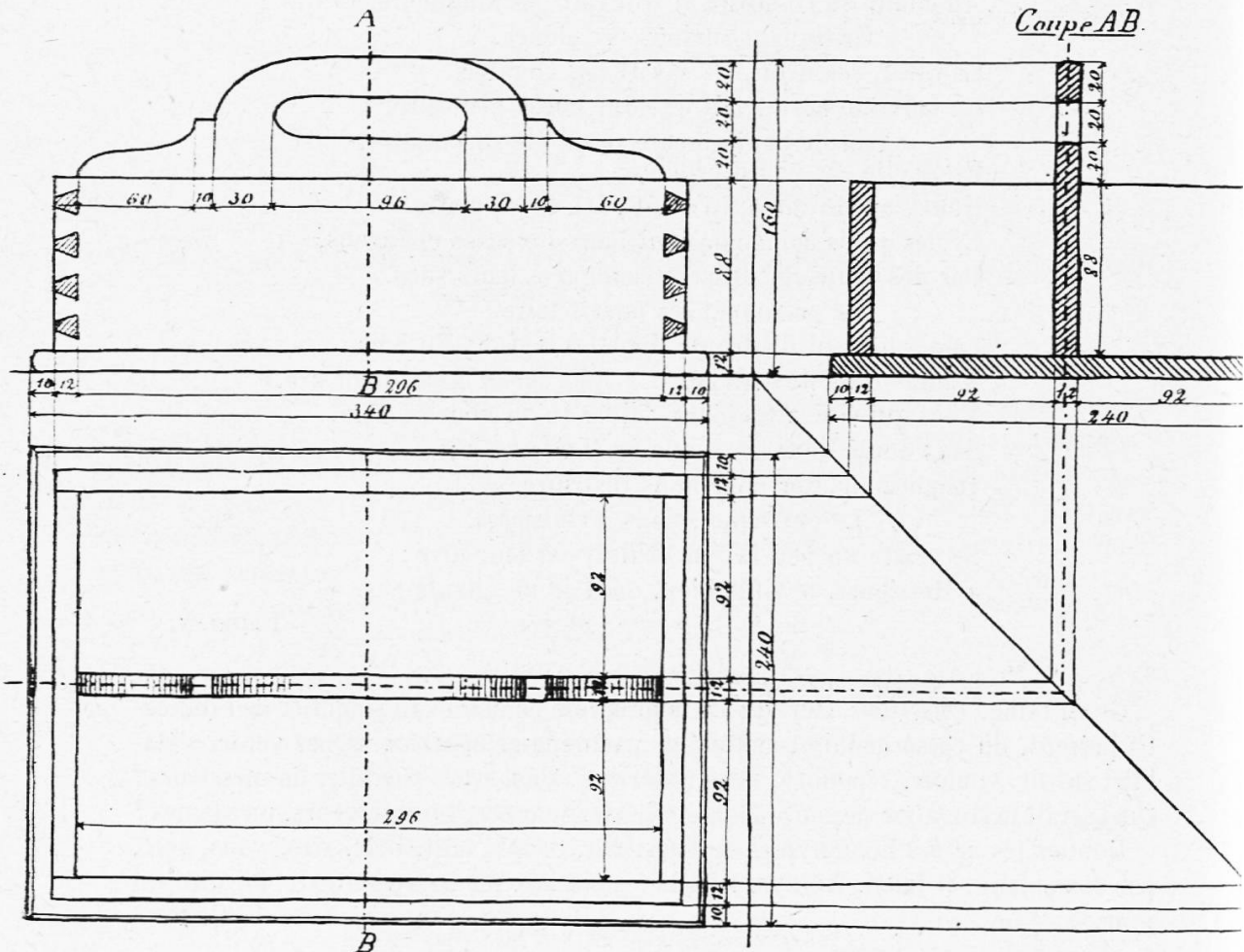
Croquis coté d'une boîte à clous à 2 compartiments.
