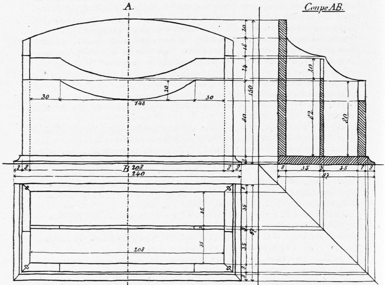
Croquis coté d'un porte-cartes.
