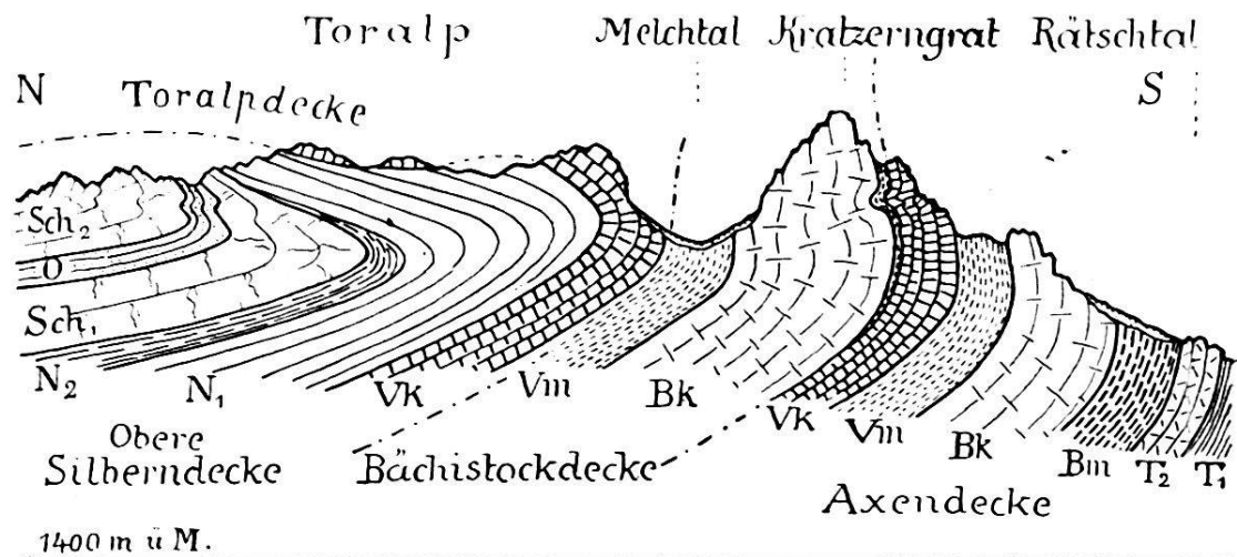
FIG. 1. — Profil durch Toralalp und Kratzergrat.
