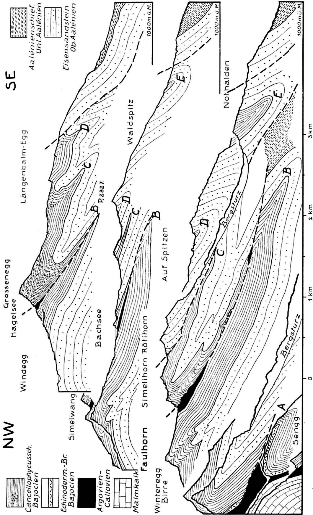
Fig. 2. Die südlichen Doggermassen der W-Faulhorngruppe von H. Günzler-Seiffert.
