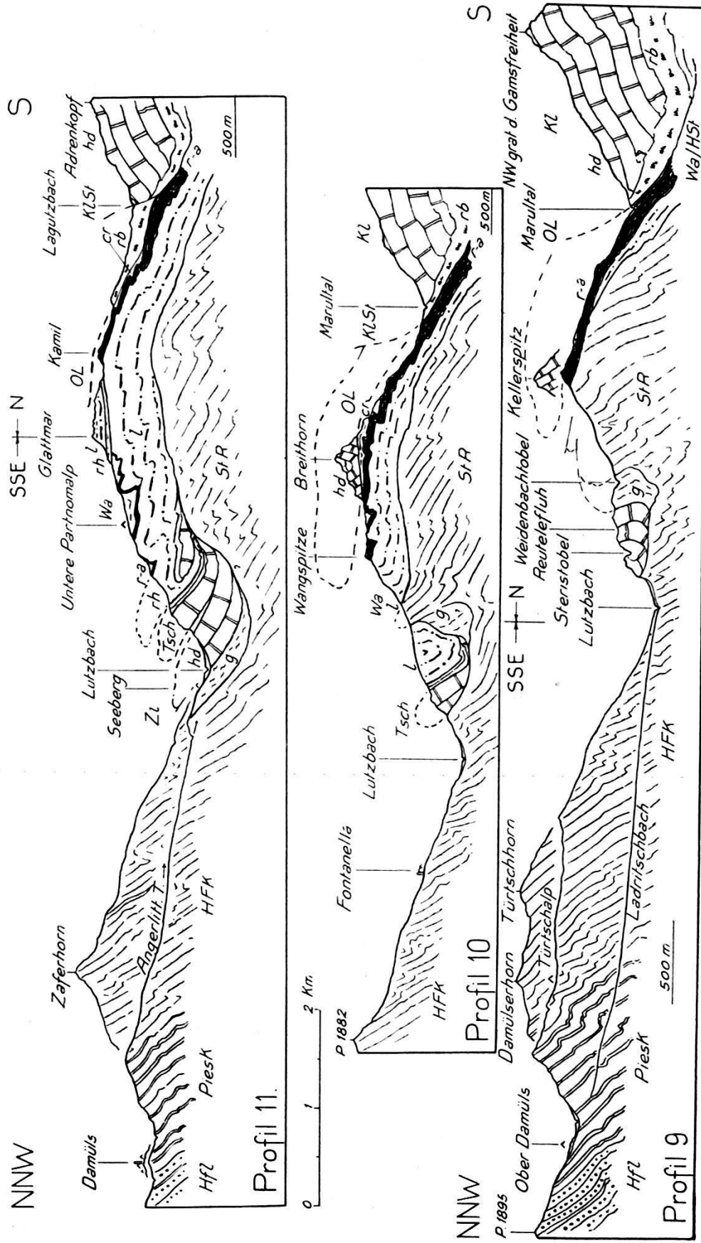
Fig. 3. Profilsérie durch das Westende der Allgäu-Decke. (Grosses Walsertal-Marulltal.)
