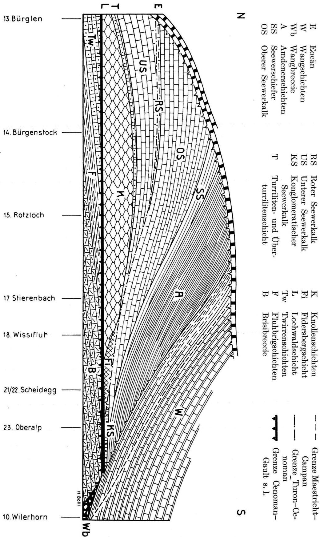
Fig. 6. Schematischer Querschnitt durch die Entwicklung der Oberkreide im abgewinkelten Ablagerungsraum der höheren helvetischen Decken.
