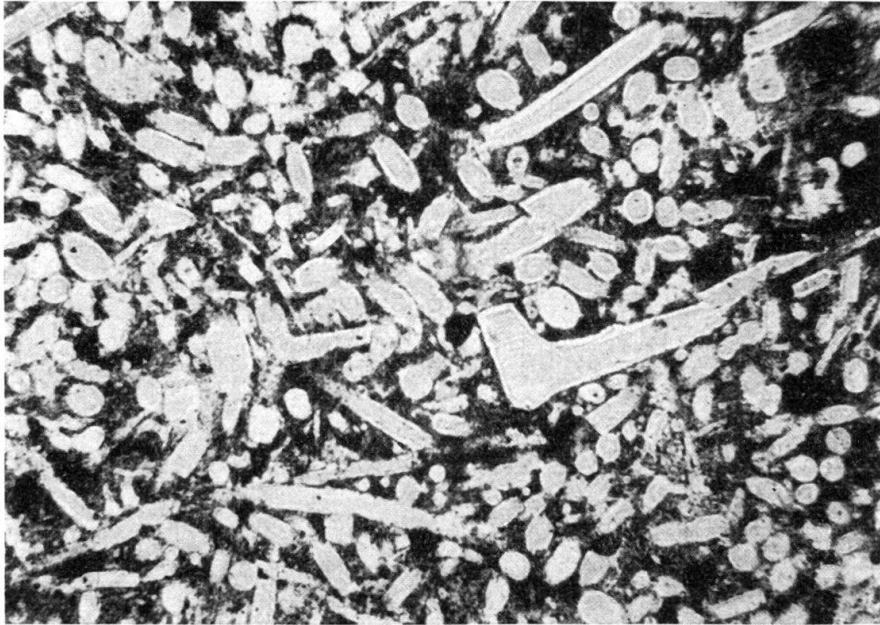
Fig. 4. Galet L 10, station de Baumaroche II. Spongolithe ; spicules calcédonieux dans une gangue calcaréo-cherteuse. 36:1, lumière naturelle.
