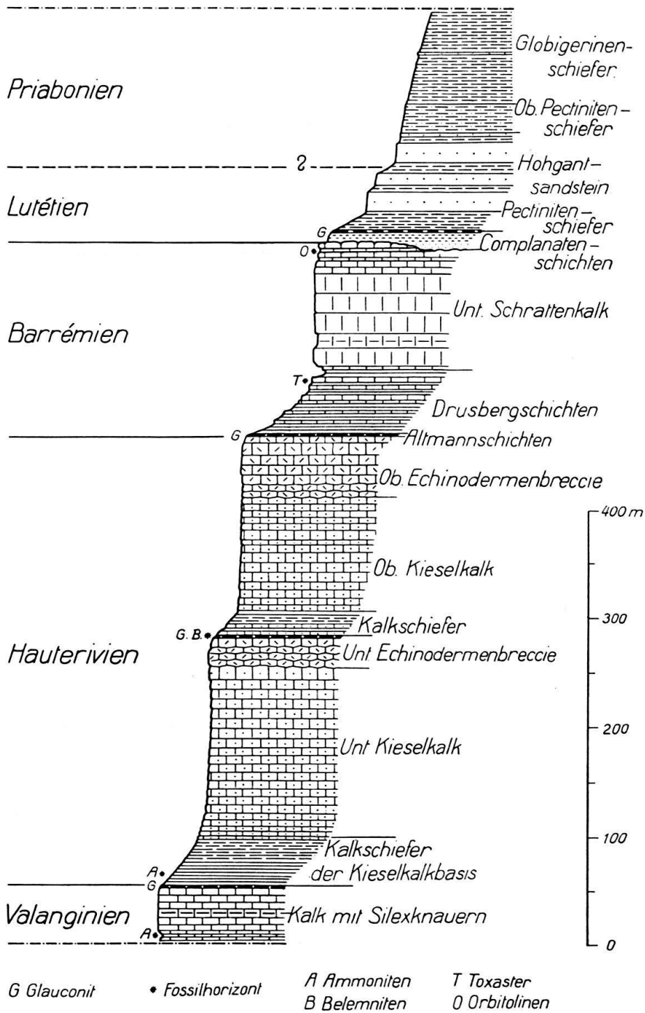
Fig. 2. Stratigraphisches Sammelprofil durch die Randkette im Abschnitt der Schwändeliflugh.
