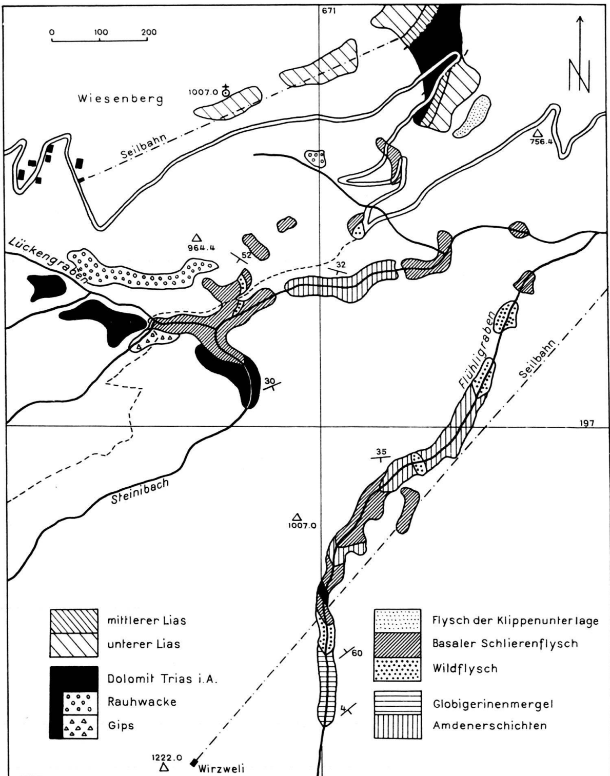
Fig. 6. Detailskizze des Flühligrabens und des unteren Steinibaches
