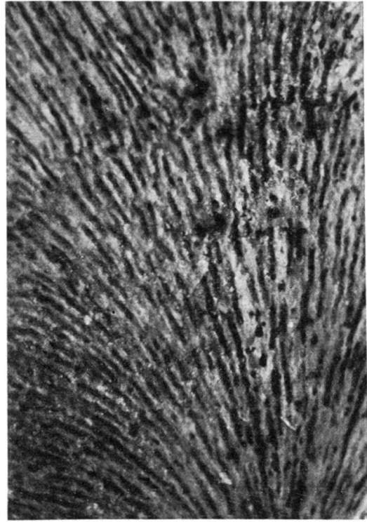
Fig. 24. Emscheria firma sp. nov. Surf. pol'e radiale. Holotype. Gross. environ 8 fois
