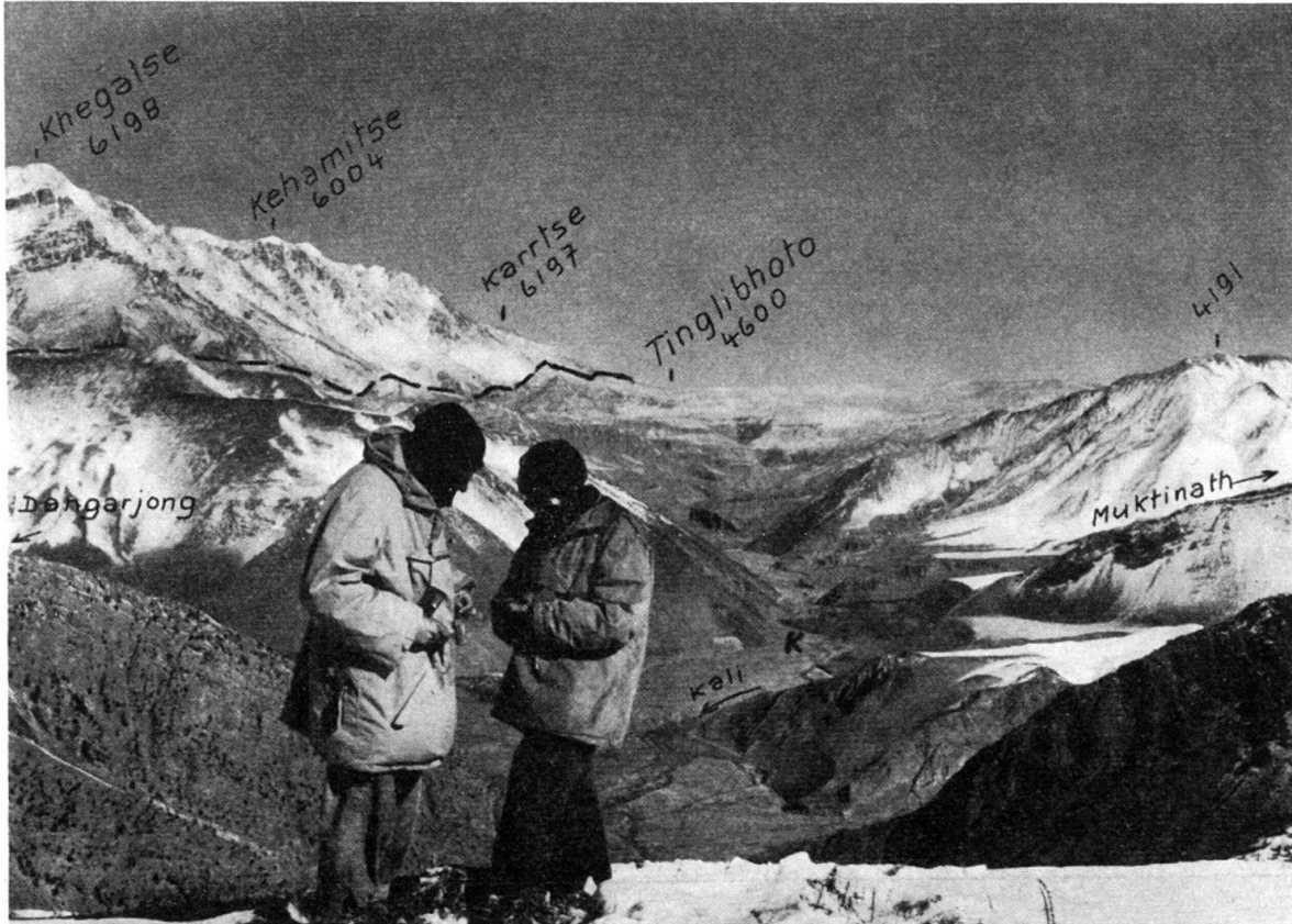
Fig. 5. Der Thakkhola Graben von Süden gesehen. Die gestrichelte Linie bezeichnet die Dhangarjong-Verwerfung. Westlich der genannten Verwerfung (im Bilde links) stehen silurisch-devonische Schichten an, welche den Unterbau des Khegatse und des Kehamitse bilden. Östlich der Verwerfung finden sich die obermesozoisch-tertiären Schichten der Thakkholaserie. Diese fallen stark nach Westen, wie unter Pt. 4191 deutlich zu sehen ist. – Im Talhintergrund die flache Wasserscheide zum Tsangpo.
