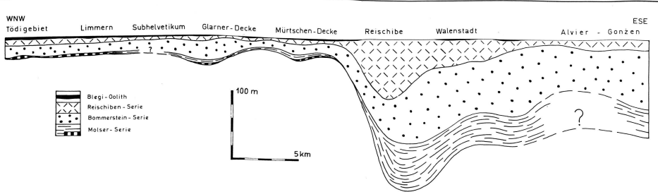
b. Schematische Abwicklung der Doggerserien zwischen Linth und Rhein
