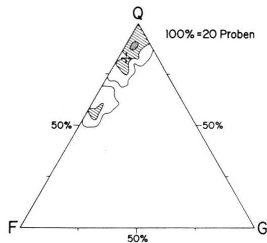
f) Subalpiner Flysch
